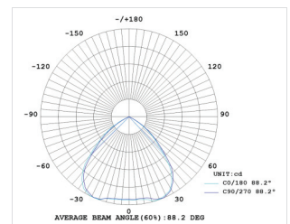
90° Reflector
